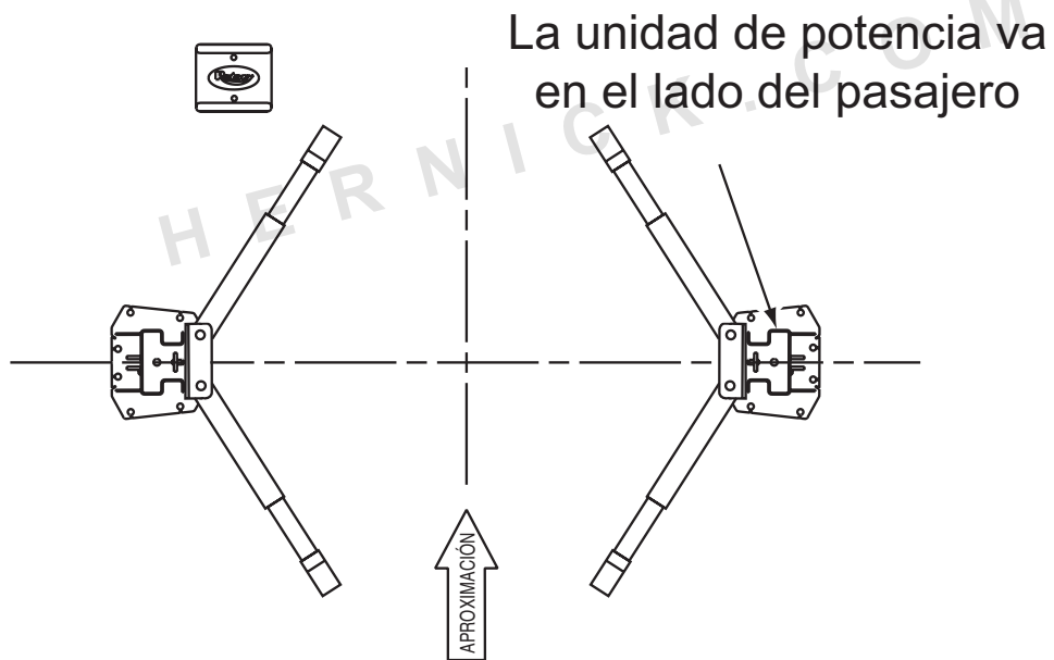
SPO10 Vista de planta
