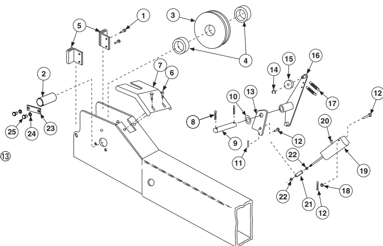
DETALLE DEL EXTREMO DEL YUGO TRASERO
